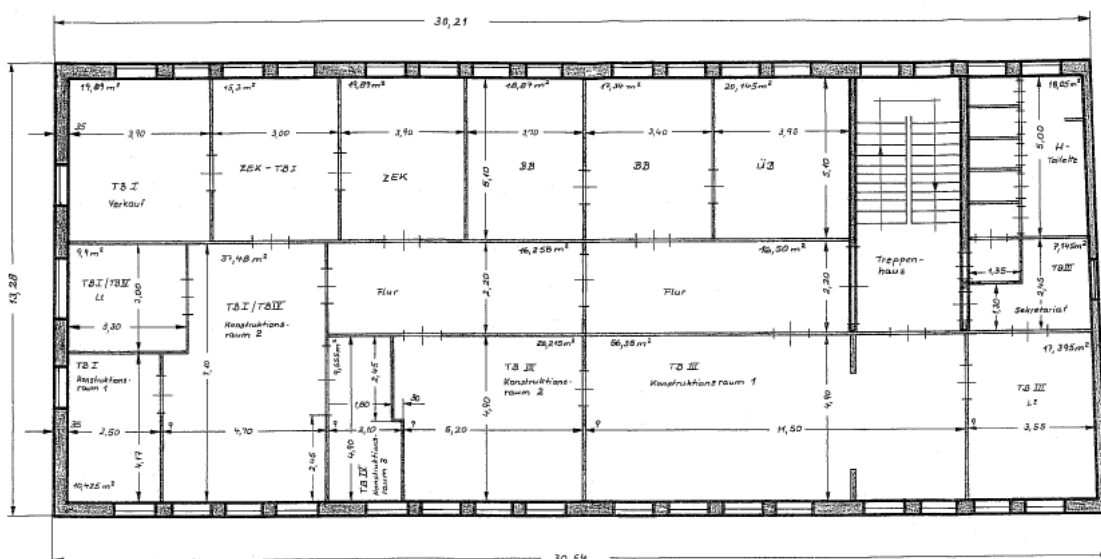
Grundriss des 1. OG
